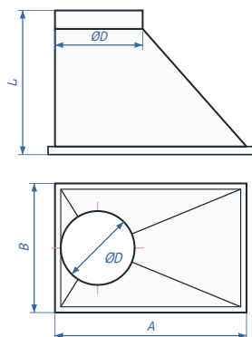
Тип-4 \varnothing D / A \times B - L - тип4
