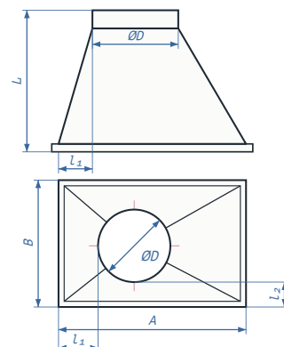
Тип-6 \varnothing D / A \times B - L - l_1 - l_2 - тип6
