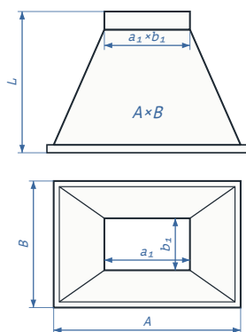
Тип-1 A \times B / a_1 \times b_1 - L
