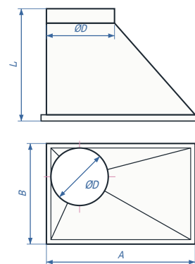
Тип-3 \varnothing D / A \times B - L - тип3
