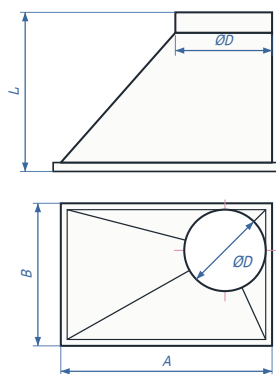
Тип-2 \varnothing D / A \times B - L - тип2
