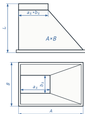
Тип-4 A \times B / a_1 \times b_1 - L - тип4
