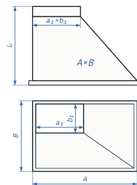
Тип-3 A \times B / a_1 \times b_1 - L - тип3
