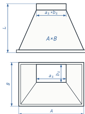
Тип-5 A \times B / a_1 \times b_1 - L - тип5
