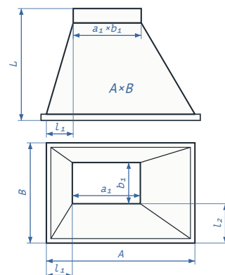
Тип-6 A \times B / a_1 \times b_1 - L - l_1 - l_2 - тип6
