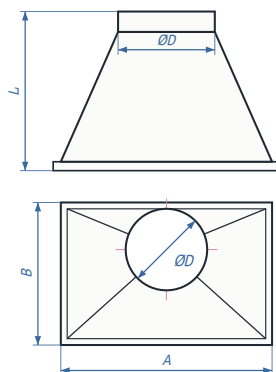
Тип-5 \varnothing D / A \times B - L - тип5
